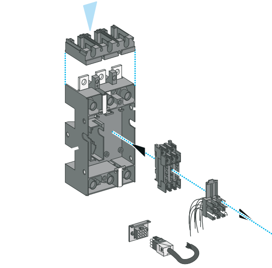
Mühürlenebilir terminal koruyucuları
